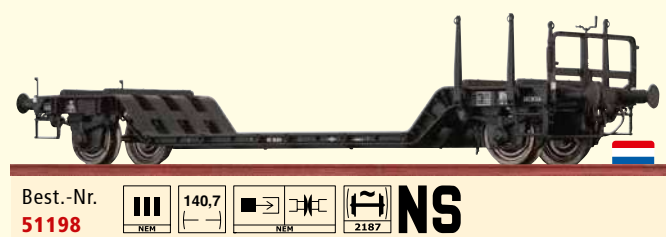
Tiefladewagen Ui NS Betriebs-Nr. 21 84 909 1 000-8
