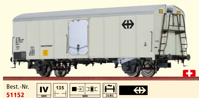
Kühlwagen Ibps-v SBB Betriebs-Nr. 42 85 805 7 010-2
